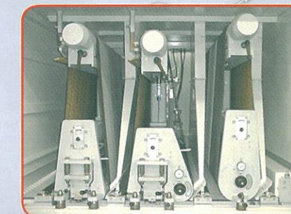
Optie: schuurband- lengte 2620 mm
